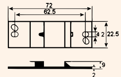
ASYMMETRICAL DIN ADAPTOR - A
