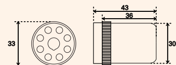
FREE SOCKET - 8 pole US-08 - 11 pole US-11
